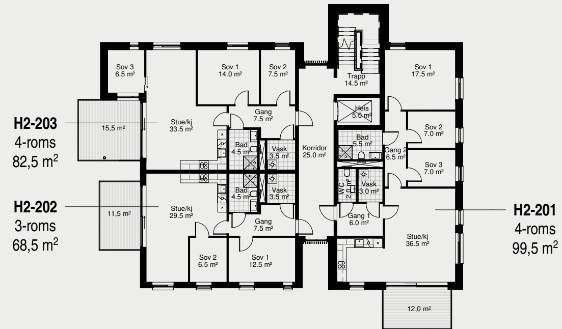
HUS 2 | 2. ETASJE
