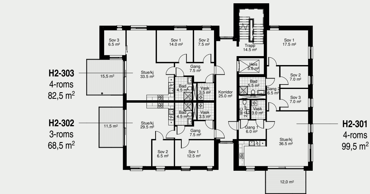
HUS 2 | 3. ETASJE
