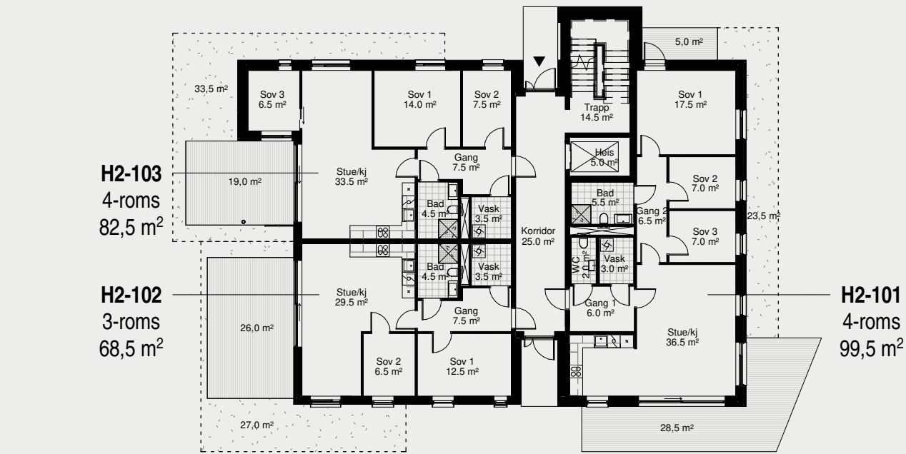
HUS 2 | 1. ETASJE
